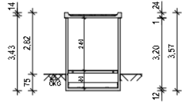
Schnitt M 1 : 100
