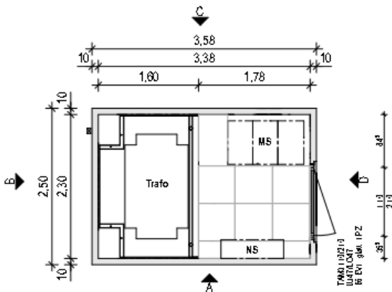
Grundriss M 1 : 50
